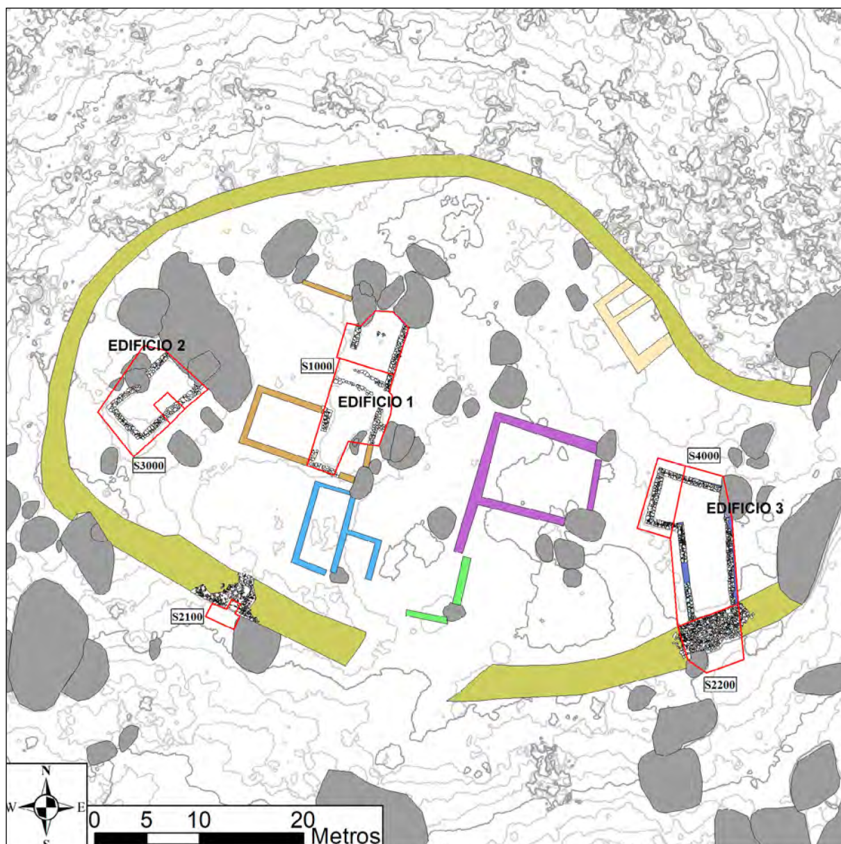
Figura 3. Plano del yacimiento con indicación de los sectores y edificios excavados (elaboración propia).
